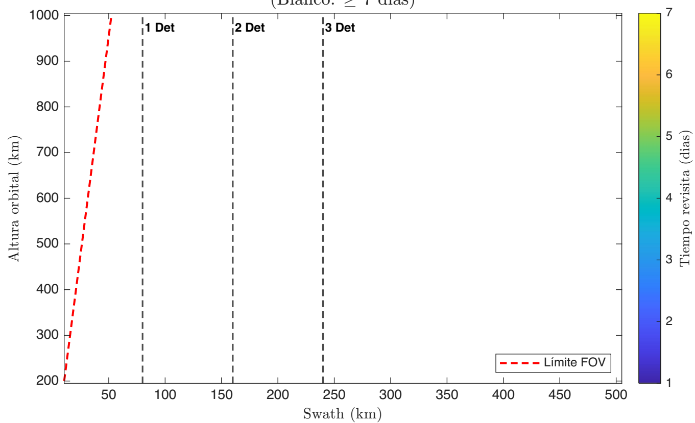
Tiempo Revisita - 1 Satellite(s); 1 Telescopio(s): Cassegrain; Detector 3 (Blanco: \geq 7 dias)
